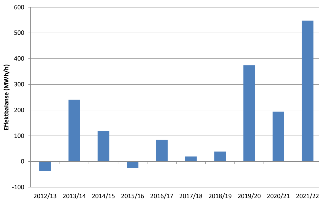
Figur 8 Historisk effektbalanse i tunglasttime – målte verdier
